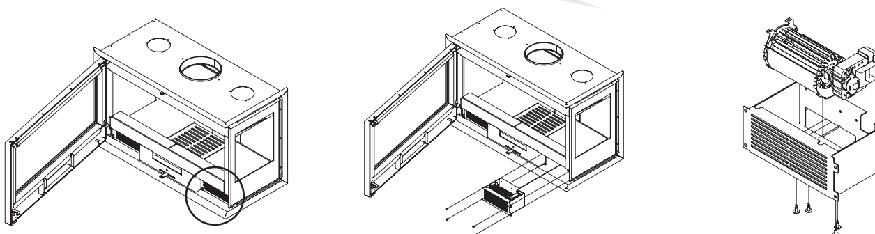
Sostituzione delle turbine degli inseribili F e PANORAMIC
