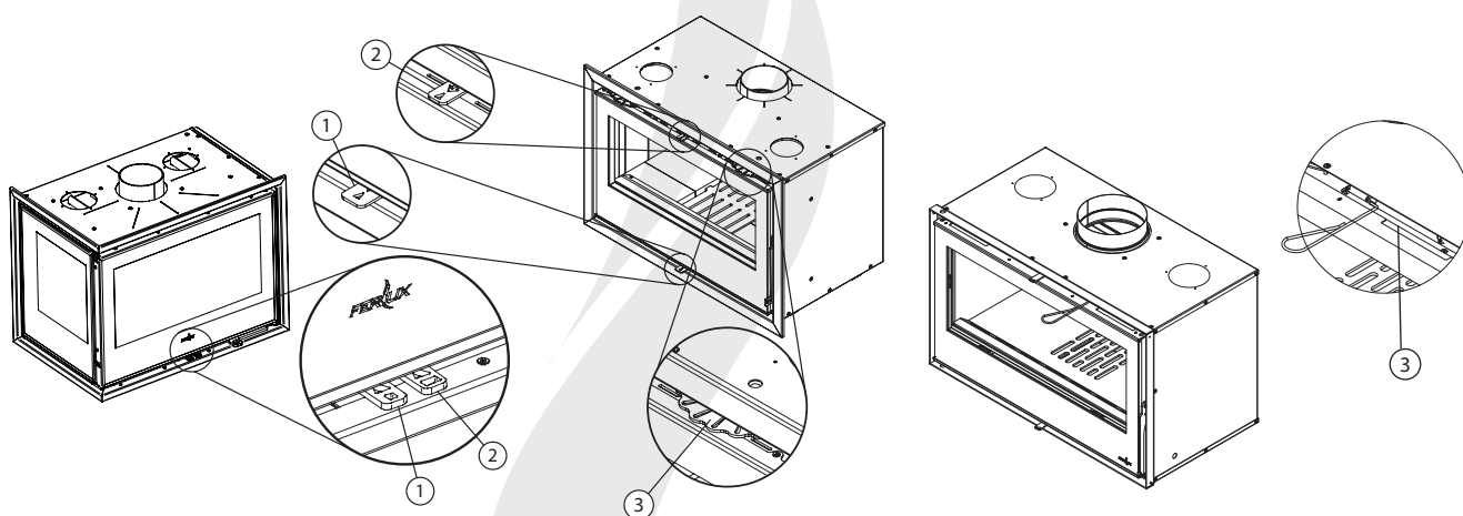
Comandi dell'apparecchio (PANORAMIC a sinistra, GALAXY/TAURUS al centro e F-TEIDE a destra)
