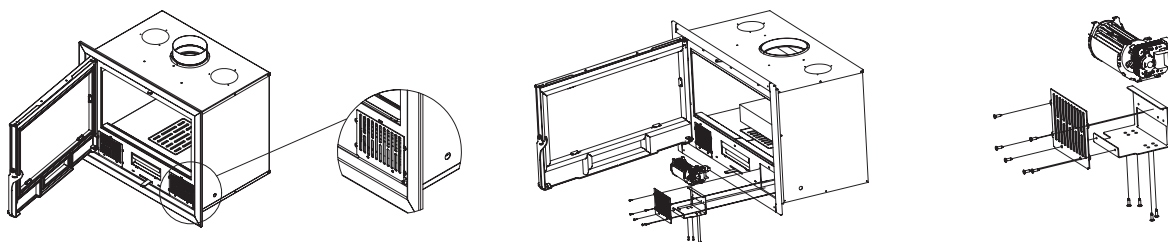
Sustitución de las turbinas en los insertables FUJI/TEIDE
