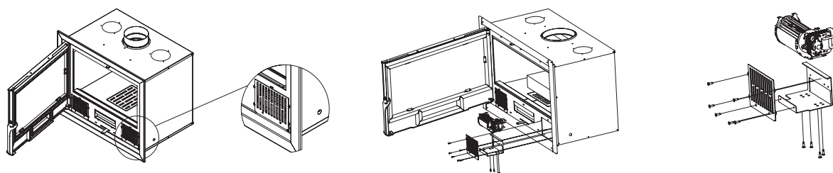
Substituição das turbinas nos encastráveis FUJI/TEIDE
