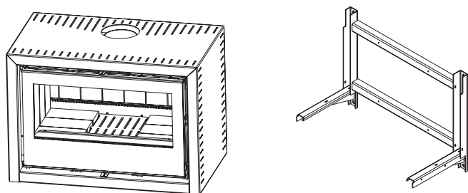
GALAXY MINIMAL y estructura de soporte a pared GALAXY MINIMAL e estrutura de suporte à parede GALAXY MINIMAL and wall support structure GALAXY MINIMAL e struttura di supporto a parete
