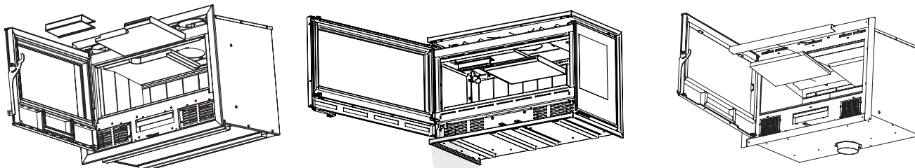
Desmontagem do defletor de vermiculite nos aparelhos GALAXY/TAURUS , PANORAMIC e TEIDE/FUJI
