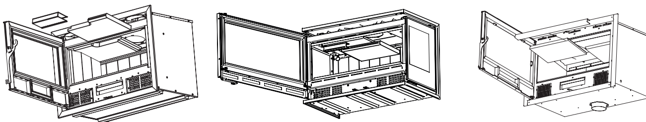
Smontaggio del deflettore su apparecchi GALAXY/TAURUS - PANORAMIC - FUJI/TEIDE
