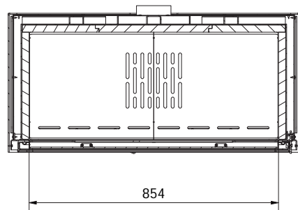
D-D ( 1 : 10 )
