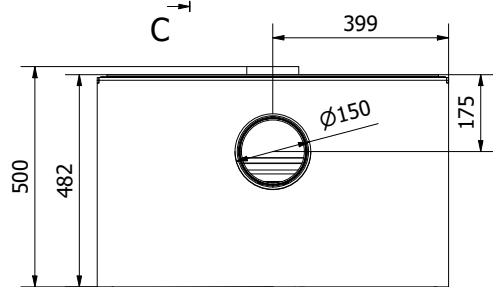
D-D ( 1 : 10 )
