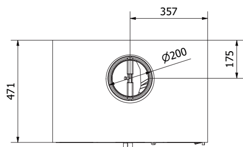
G-G ( 1 : 10 )
